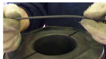
Fig. 38 Déposer le joint torique (412.1) du bol (157).
