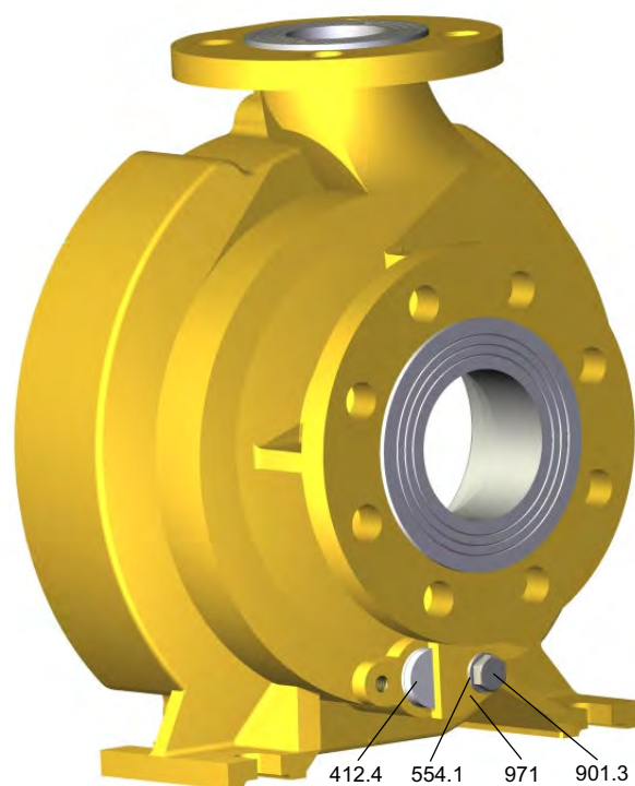
Fig. 26 Dessin d'exécution spéciale UTN-BL avec corps drainé (voir le Tableau des codes DIN à la page précédente).
