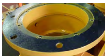
Fig. 40 Démontez la bride du moteur (347) de la lanterne (344) en dévissant les vis prévues à cet effet.
