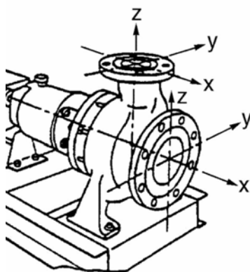
Fig. 22 Forces et moments. Axe x: aspiration, Axe z: refoulement.
