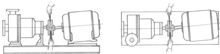
Fig. 17 Angulaire : le défaut d'alignement maximum autorisé est de 0,8 mm (pour un raccord de 96 millimètres de diamètre).
