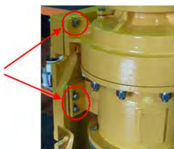
Fig. 59 Installer la pompe sur le moteur à l'aide d'un engin de levage approprié. Visser le moteur sur la lanterne (344) verticale. Fig. 60 Pour un montage pratique, maintenir la pompe à la verticale. Serrer les vis pour fixer le châssis (891) à la pompe. avec les vis prévues à cet effet.
