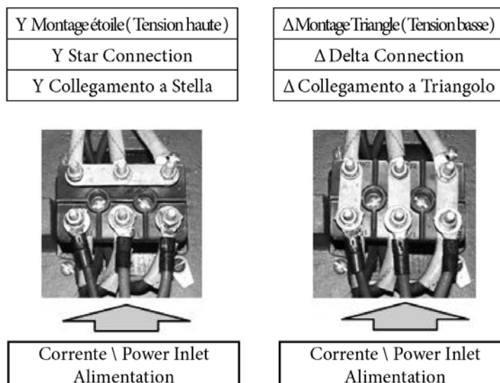
Fig. 20 Les connexions électriques du moteur.
