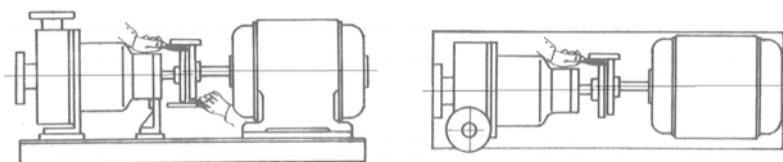
Fig. 18 Latéral : un léger décalage parallèle ne dépassant pas 0,2 mm peut être toléré avec ce type de raccords.
