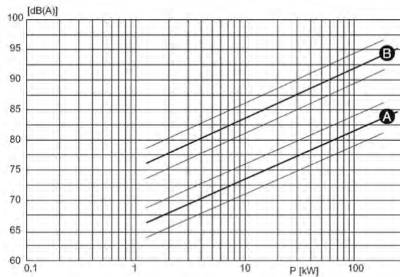
Fig. 8 Graphique relatif au niveau sonore à l'échelle logarithmique.
