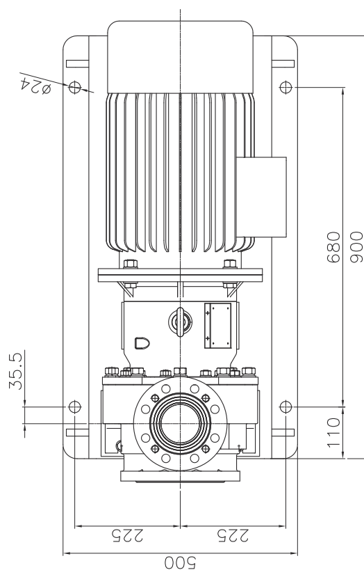
Fig. 62 Schéma d'encombrement UTN-BL 125-80-160 Mot. B5.
