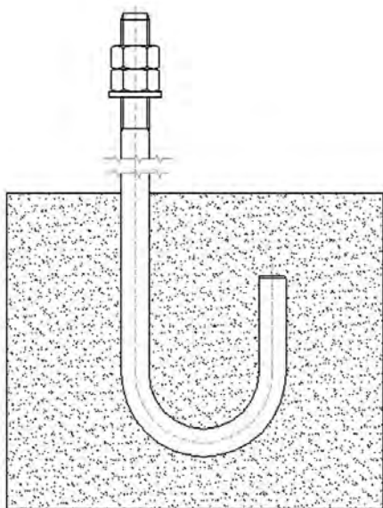
Fig. 13 Fondations pour la fixation du groupe pompe moteur.
