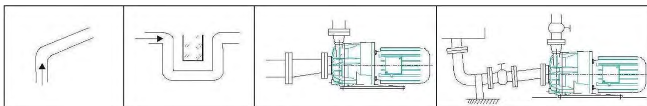
Fig. 15 Installation recommandée de la tuyauterie d'aspiration.
