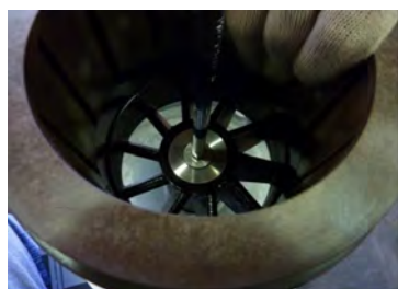
Fig. 30 Dévisser la vis (918) pour démonter le coupleur magnétique externe (102) de la lanterne (344) en dévissant les écrous prévus à cet effet.
