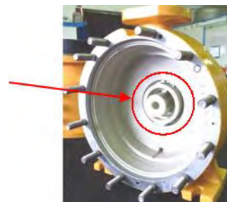
Fig. 32 Extraire le corps aspirant (106) du corps de pompe (102) en soumettant le corps aspirant (106) à une rotation dans le sens contraire des aiguilles d'une montre.
