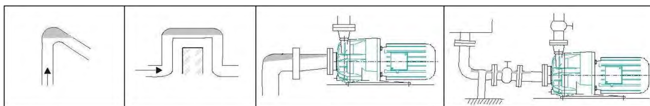
Fig. 16 Installation déconseillée de la tuyauterie d'aspiration.
