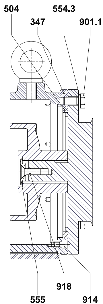
Fig. 24 Section générique UTN-BL pour l'application à un moteur de tailles 80/90/100/112.
