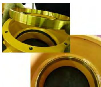
Fig. 44 Poser l'anneau anti-étincelles (516) dans son siège à l'intérieur de la lanterne (344).
