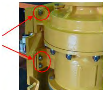
Fig. 27 Pour un démontage pratique, placer la pompe à la verticale. Dévisser les écrous et dégager le châssis (891) du reste de la pompe.
