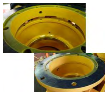
Fig. 49 Accoupler la bride d'adaptation moteur (347) à la lanterne (344) et serrer les vis.
